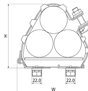
DOPPELTER, FIXIERTER DREHFUSS: ER55-62 BIS ER119-128
